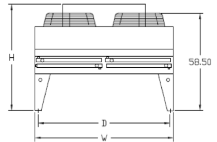
END VIEW FEV*25, FEV*26, FEV*27
